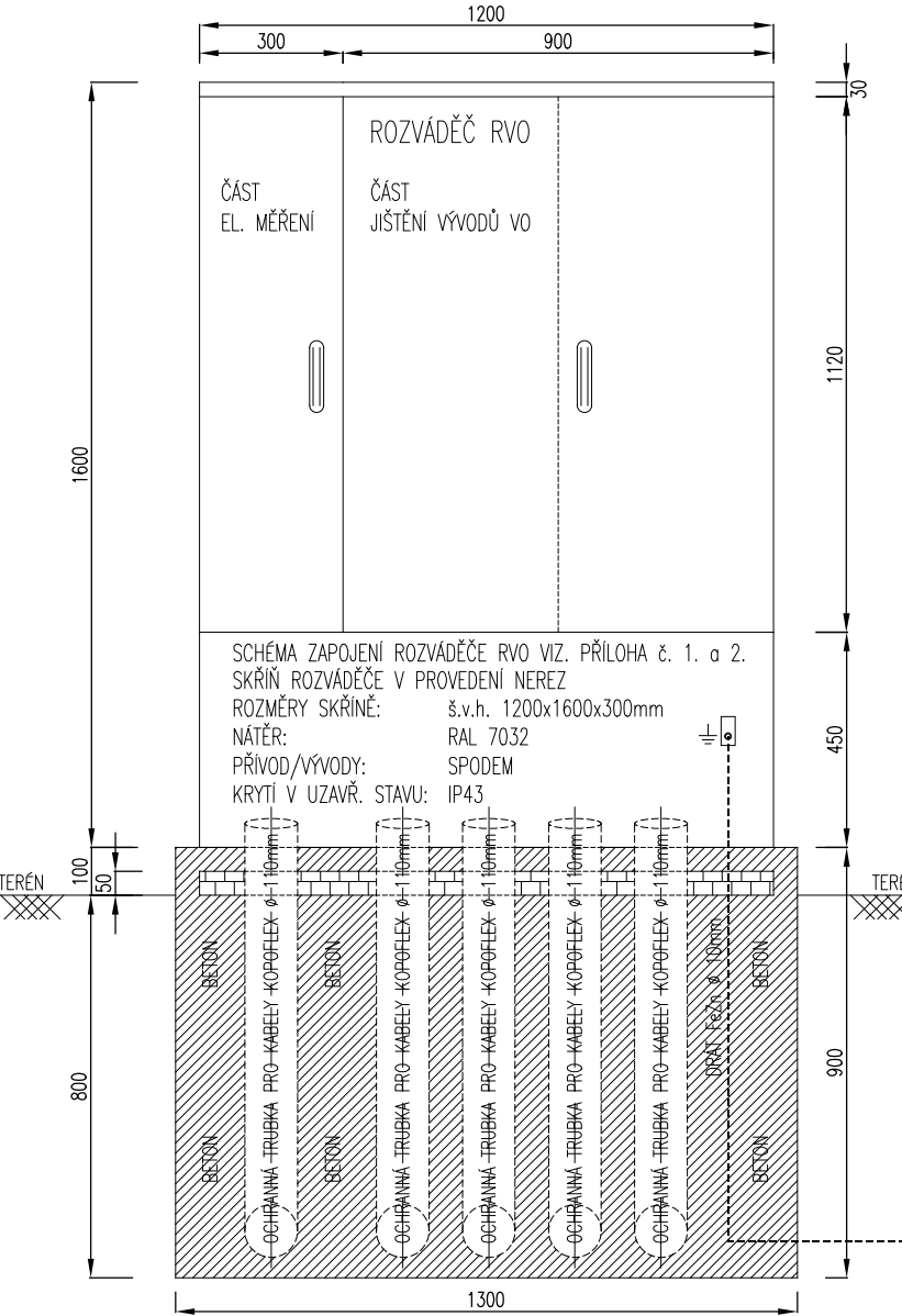
POHLED – ČELNÍ / ŘEZ
