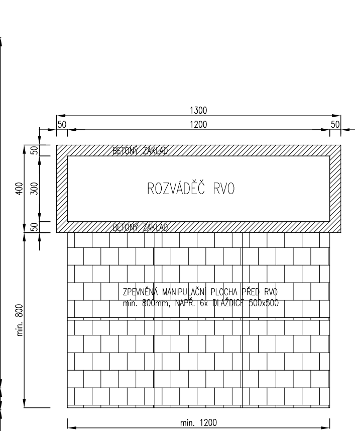
PŮDORYS
