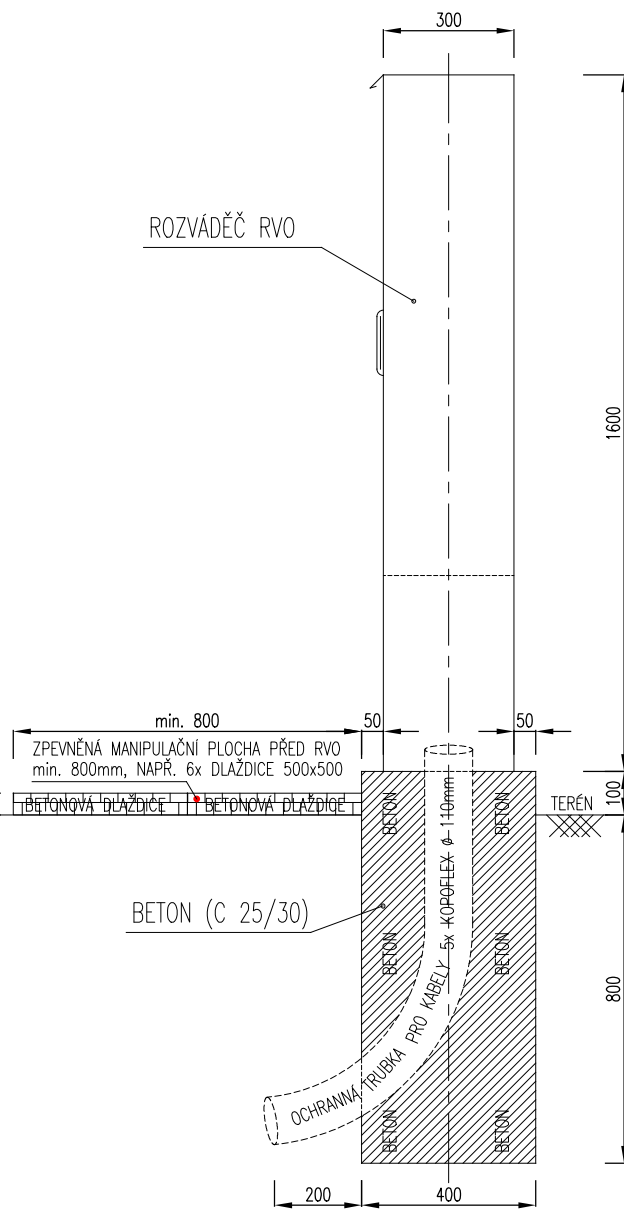
POHLED – BOČNÍ / ŘEZ
